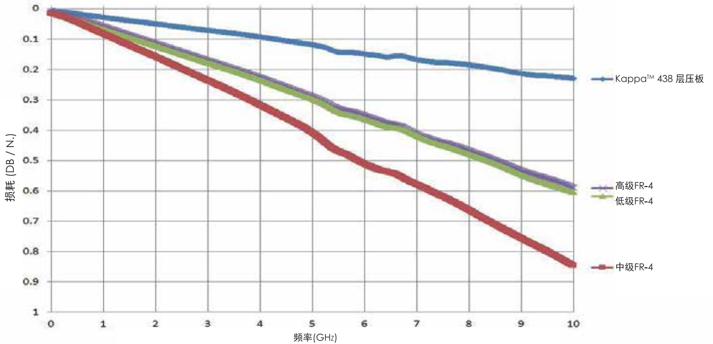
微带线插入损耗, 差分长度法, 使用30min厚度电路材料
